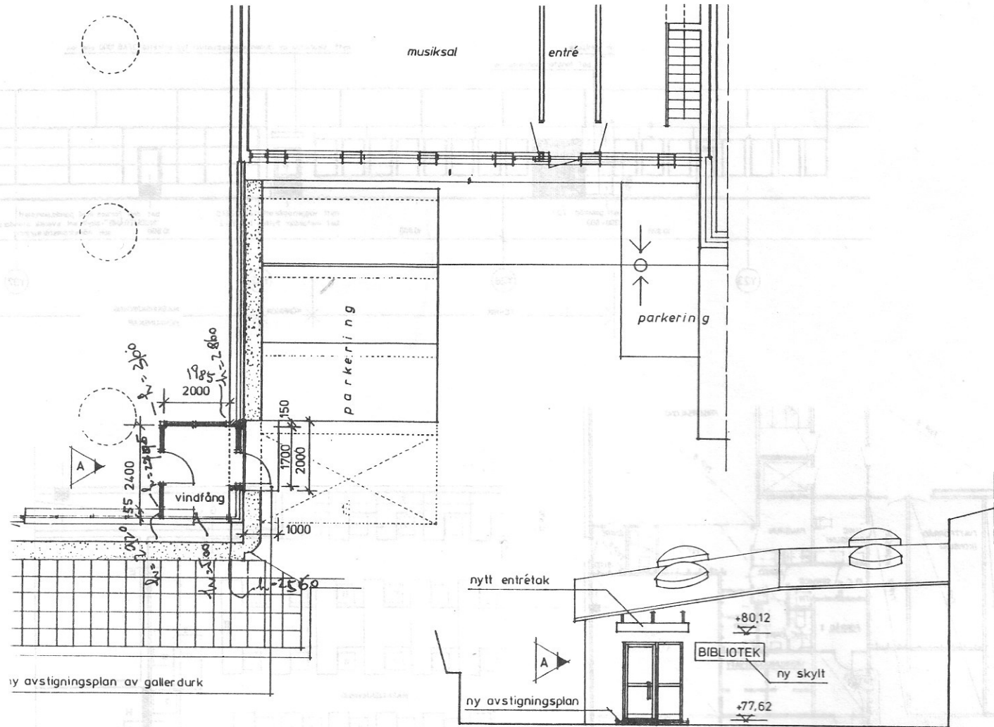
Ombyggnad av Sjumilaskolan, Göteborg, 1982; byggherre: Göteborgs skolförvaltning.
