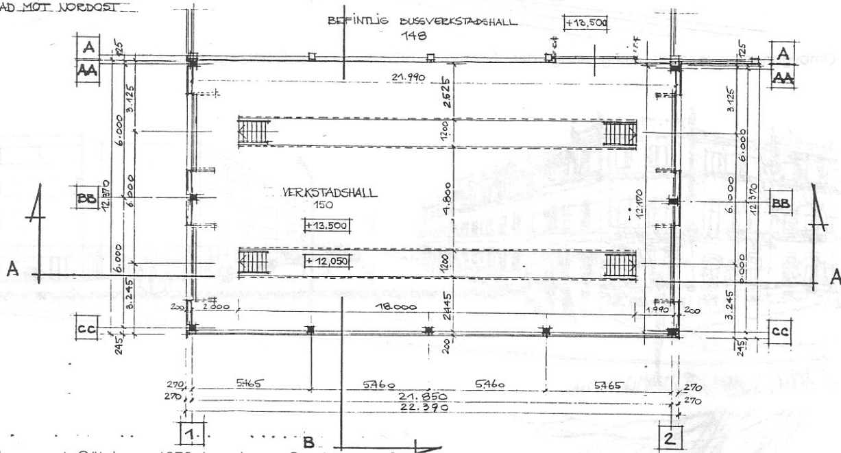
Tillbyggnad av Kvillegaraget, Göteborg, 1978; byggherre: Göteborgs spårvagnar.
